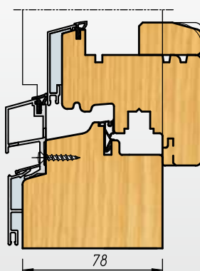
TELAIO INFERIORE ALLUMINIO TRAVERSO INFERIORE PASSANTE
