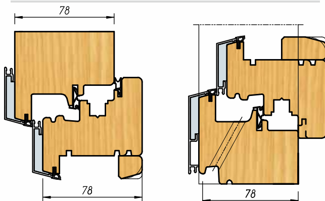
TELAIO CON CAMERA
