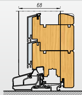
PORTA BALCONE TAGLIO TERMICO
