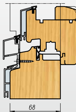
TELAIO INFERIORE ALLUMINIO TRAVERSO INFERIORE PASSANTE
