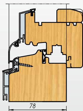
TELAIO INFERIORE ALLUMINIO CLIPS TRAVERSO INFERIORE IN LUCE
