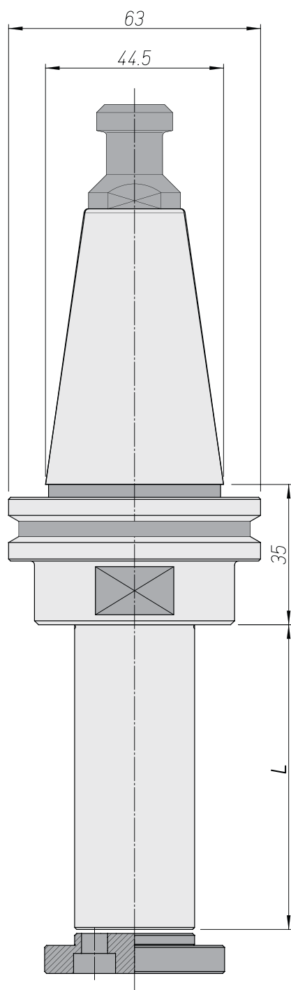
ALBERO PORTAFRESE completo di flangia e codolo
